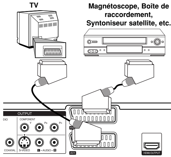
Panneau arrière du graveur
