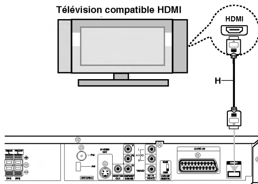
Télévision compatible HDMI
