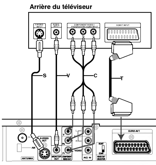
Panneau arrière du récepteur DVD/CD
