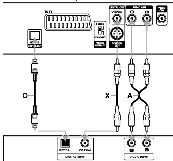
Verstärker (Receiver)
