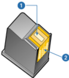
1 Gicleurs d'encre 2 Contacts en cuivre
