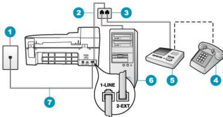
Figure 11-3 Vue arrière de l'appareil HP Tout-en-un
