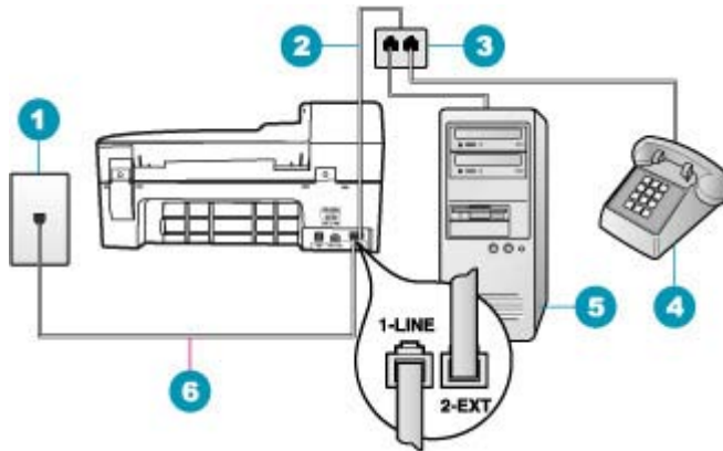
Figure 11-2 Vue arrière de l'appareil HP Tout-en-un
