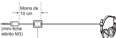
Tore magnétique - Petit (fourni)
