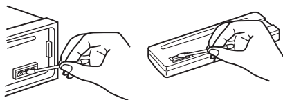
Unità principale
