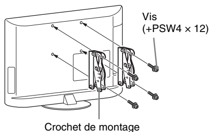
SU-WL100 (KDL-22EX310)
