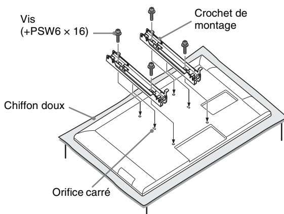
SU-WL500 (KDL-42EX410/KDL-32EX310)
