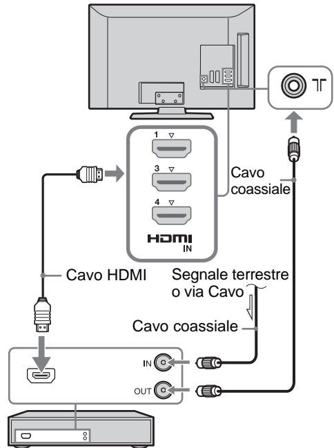
Videoregistratore/registratore DVD
