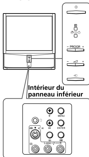
KP-ES43 Panneau avant
