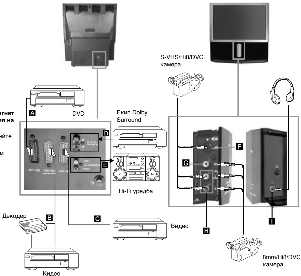
Задна страна на ретропроектора
