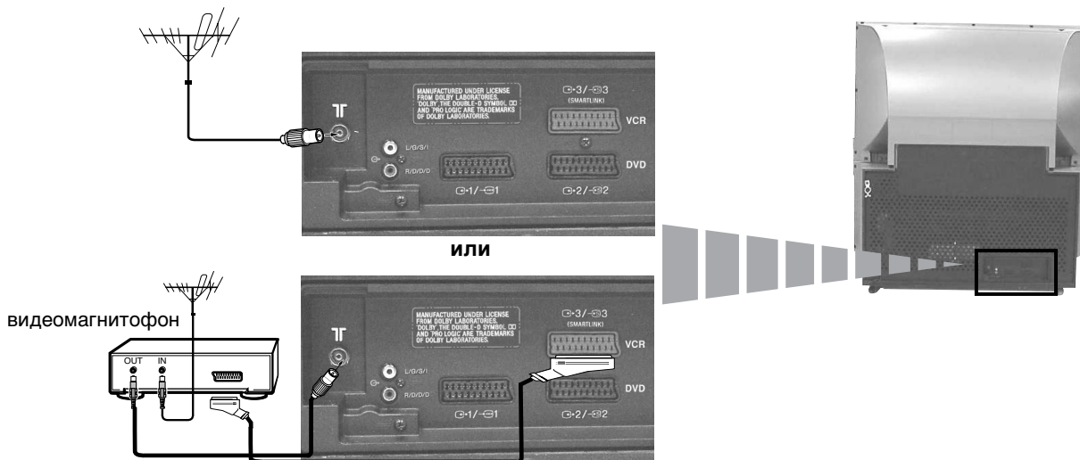
Подключение через Евроразъем (SCART) (поставляется дополнительно).
