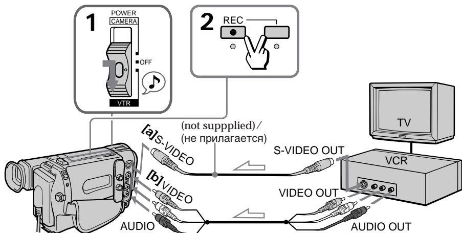
▸ : Signal flow/Передача сигнала
