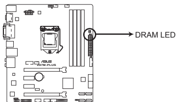
Voyant DRAM de la Z87M-PLUS
