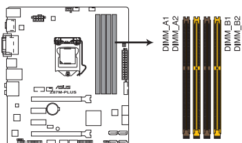
Interfaces de connexion pour modules mémoire DDR3 de la Z87M-PLUS
