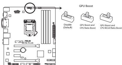
Interrupteur GPU Boost de la Z87M-PLUS
