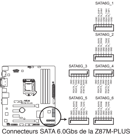
Connecteurs SATA 6.0Gbs de la Z87M-PLUS
