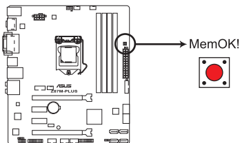
Bouton MemOK! de la Z87M-PLUS
