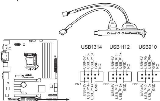
Connecteurs USB 2.0 de la Z87M-PLUS
