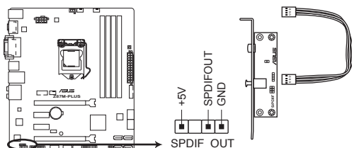
Connecteur audio numérique de la Z87M-PLUS
