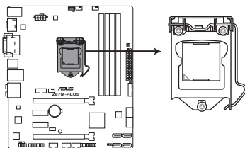
Interface de connexion LGA1150 de la Z87M-PLUS
