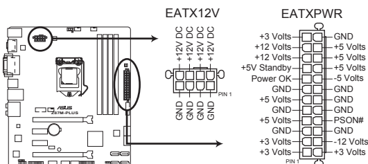
Connecteurs d'alimentation de la Z87M-PLUS
