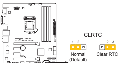
Bouton d'effacement de la mémoire CMOS de la Z87M-PLUS
