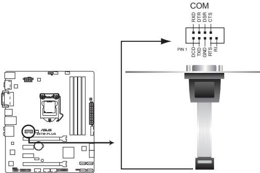
Connecteur pour port COM de la Z87M-PLUS
