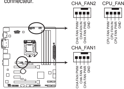
Connecteurs de ventilation de la Z87M-PLUS
