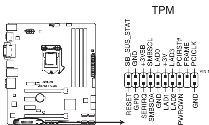
Connecteur TPM de la Z87M-PLUS
