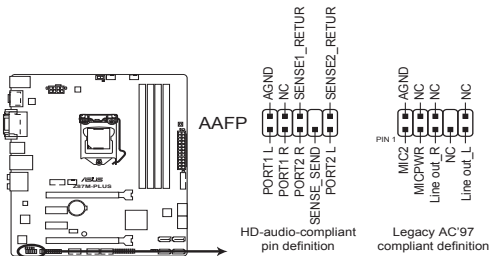
Connecteur audio pour panneau avant de la Z87M-PLUS
