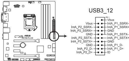
Connecteur USB 3.0 de la Z87M-PLUS
