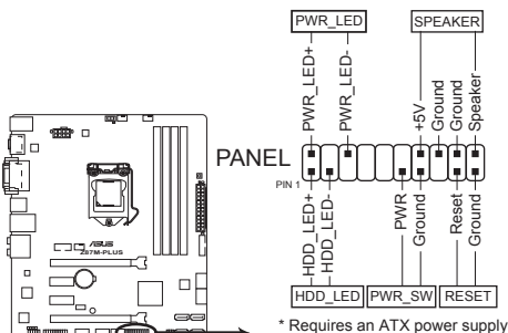
Connecteur panneau système de la Z87M-PLUS
