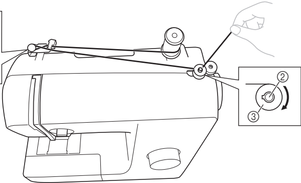
1 Disque de pré-tension 2 Axe du dévidoir 3 Canette
