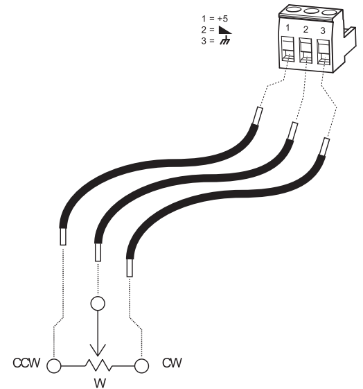
Câblage au connecteur européen à 3 broches.
