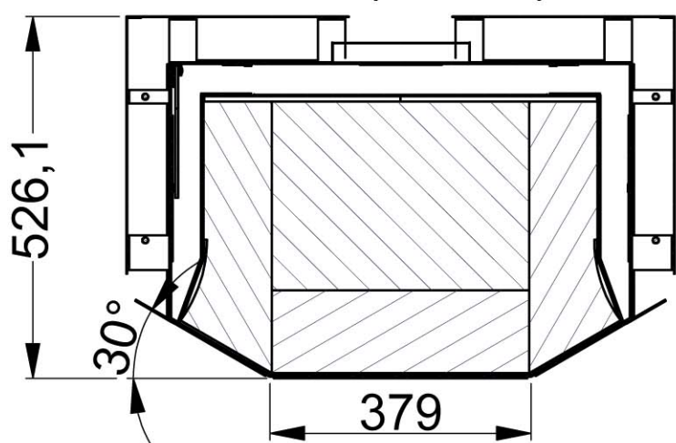
B-B ( 1 : 10 )
