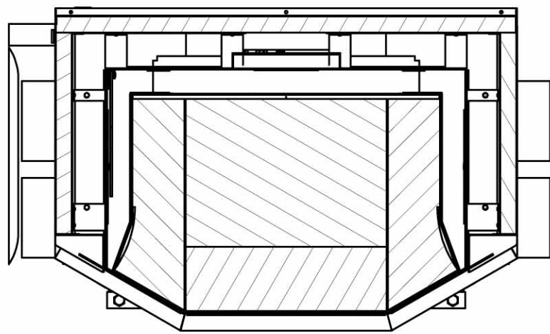
B-B ( 1 : 10 )
