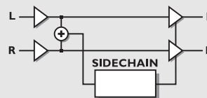
EXPANSEUR/NOISE GATE
