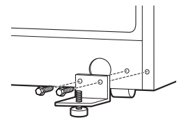
Lado derecho
