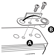
Bas de la porte du compartiment réfrigération (côté droit)
