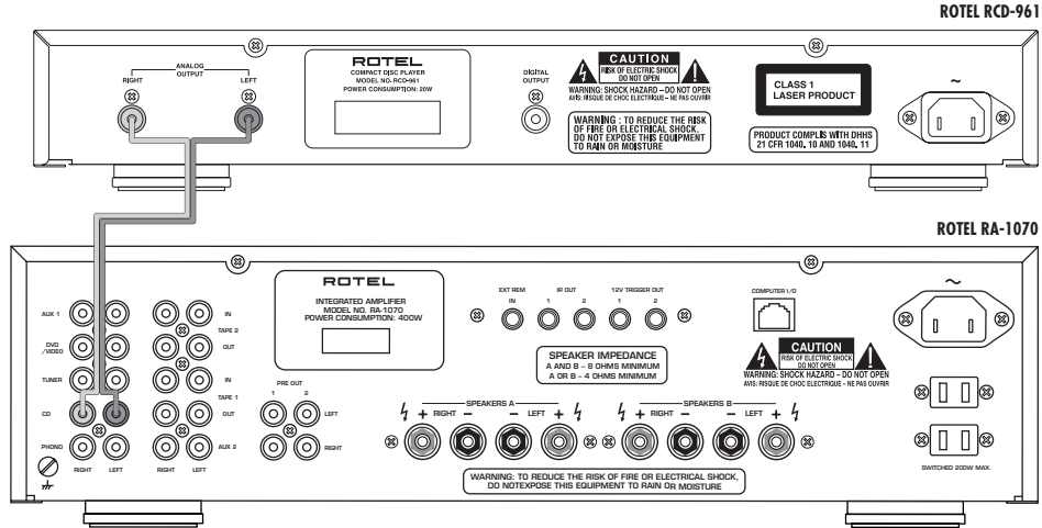
Figure 3: Analog Outputs Sorties analogiques Analoge Ausgänge Uscite Analogiche Salidas Analógicas De analoge uitgangen
