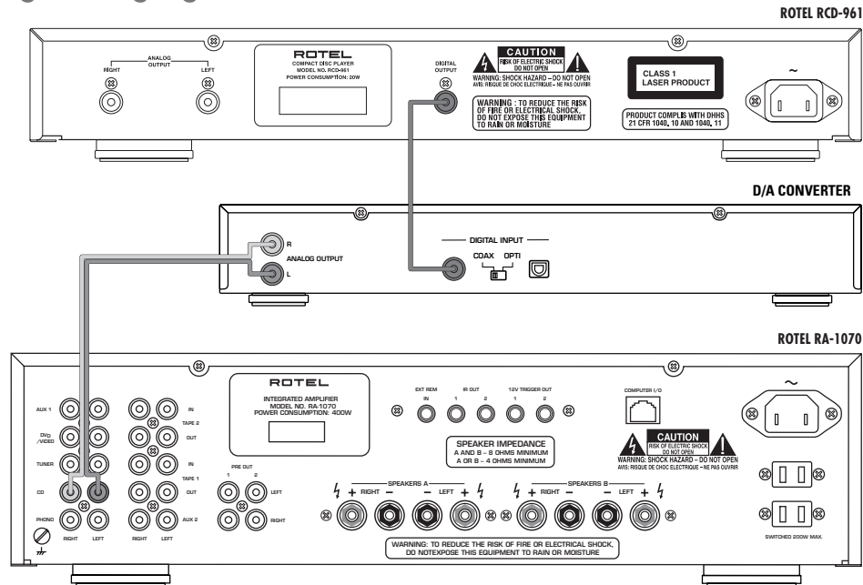
Figure 4: Digital Outputs Sorties numériques Digitalausgang Uscite Digitali Salidas Digitales De digitale uitgangen:
