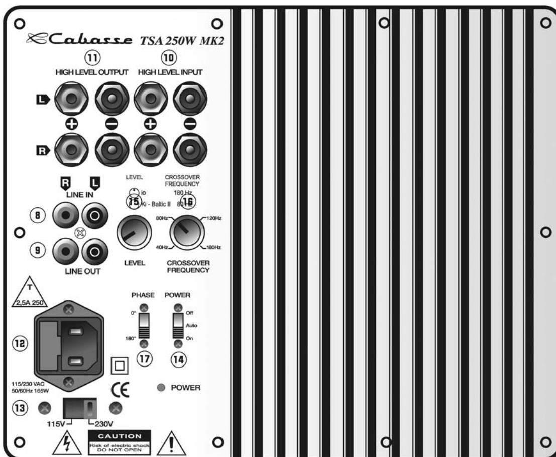
Amplificateur / Amplifier / Verstärker MERCURE
