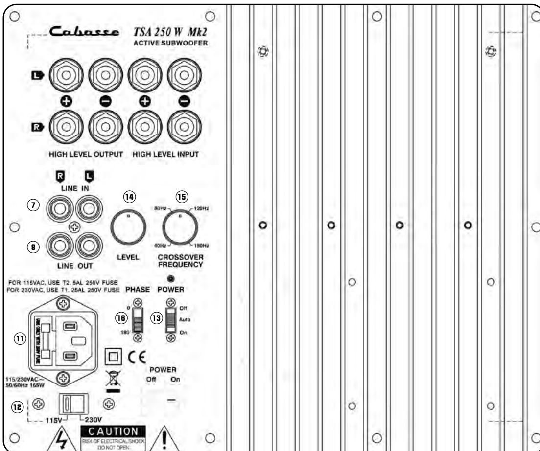
Amplificateur / Amplifier / Verstärker ORION
