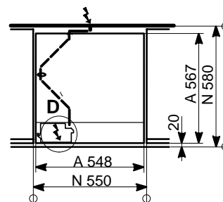
détail A
