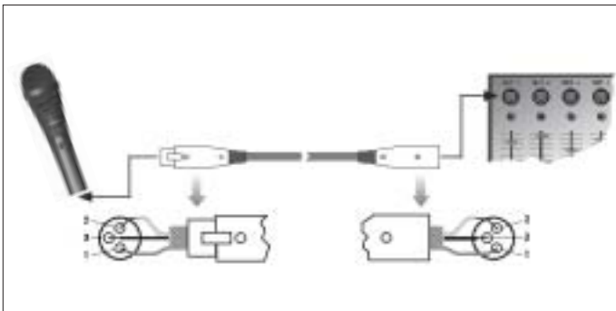
Abb. 4: Anschluss mittels symmetrischem XLR-Kabel
