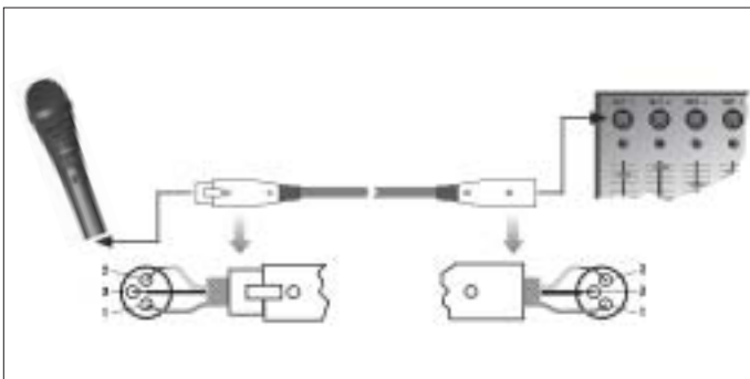
Fig. 4: Conexão através de um cabo XLR balanceado.
