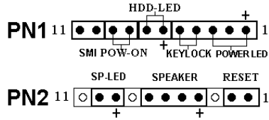
Figure 2-7. Définitions des pins des PN1 et PN2
