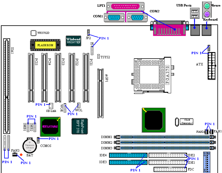
Figure 2-5. Tous les tsconnecteurs de la BX133-RAID
