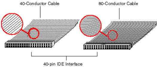
Figure 2-8. Différences entre des nappes Ultra ATA/33 et Ultra ATA/66
