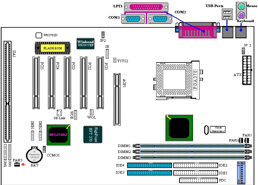
Figure 1-1. Emplacements des composants sur la carte mère
