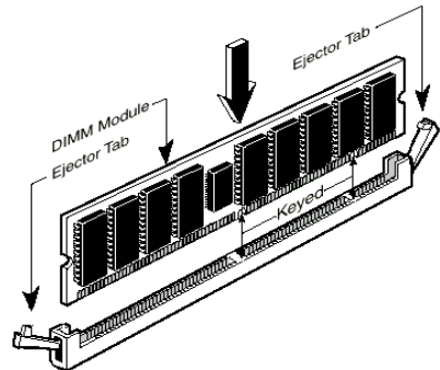
Figure 2-4. Installation du module de mémoire
