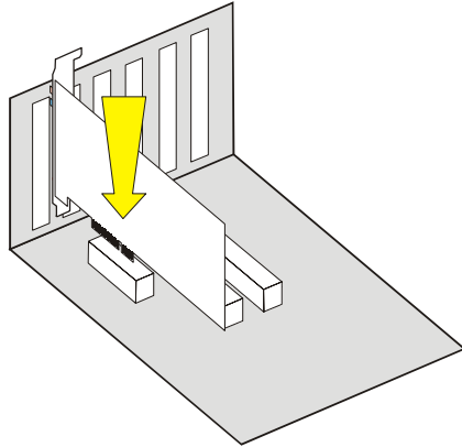
Figure 2-3. Installez la carte CNR AC11 dans le slot CNR.
