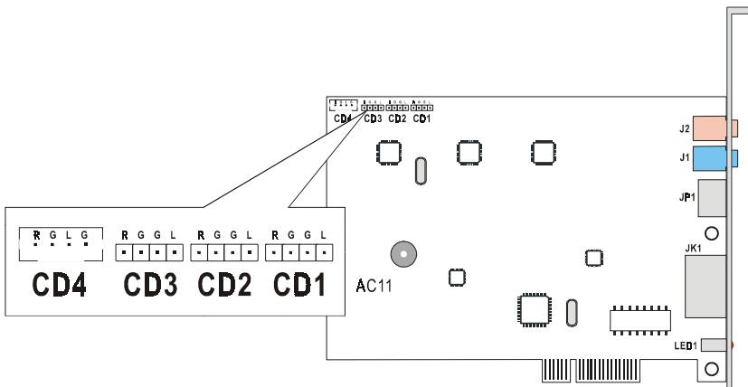
Figure 2-2. Définitions des pins des connecteurs CD1 ~ CD4.
