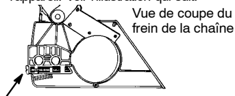
Réglage du frein de la chaîne
