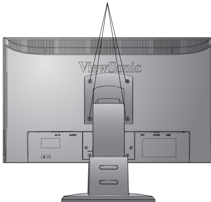
Etape 3-4. 4 vis fixant la base
