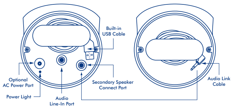
HAUT-PARLEUR PRINCIPAL
