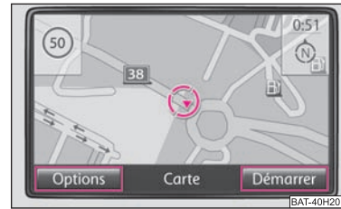
Fig. 12 Mode Cartes
