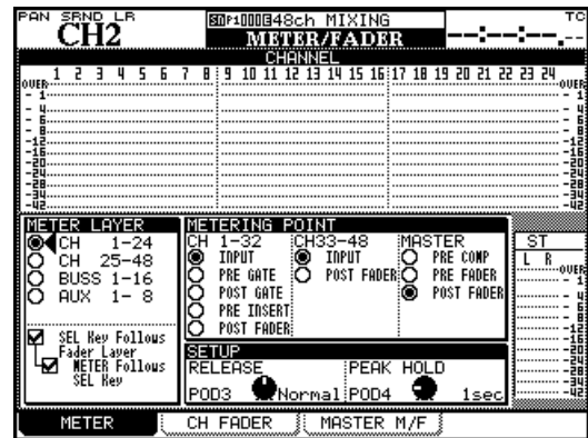
Figure 4.12: Ecran de mesure (indicateurs de niveau des 24 premiers modules de voie)
