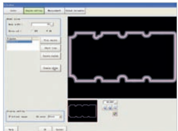
Etape 4 : calcul automatique du chemin du cordon de colle
