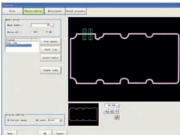
Etape 3 : définir le point de départ et de fin du cordon
