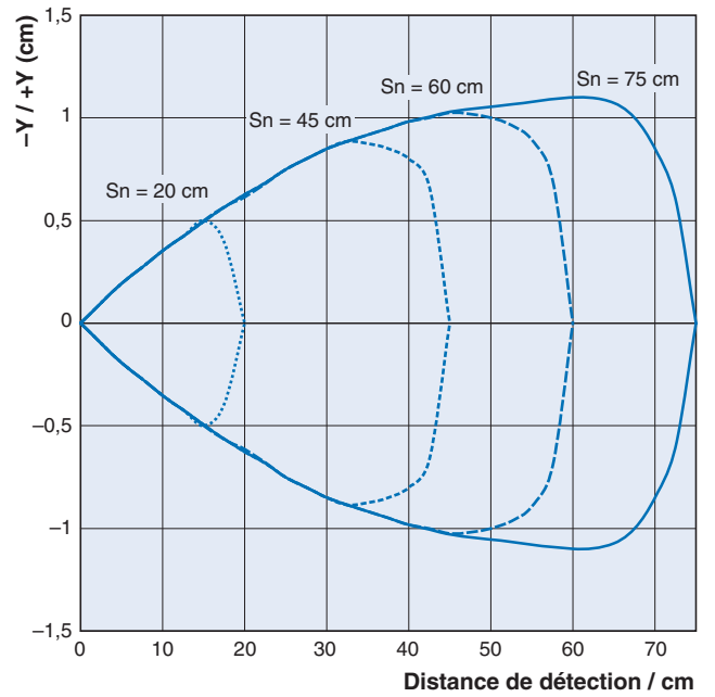
Caractéristiques d'angle du F3C, capteur pour convoyage à fonction BGS
