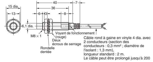
Fig. 2 : E2E-X2MY□
