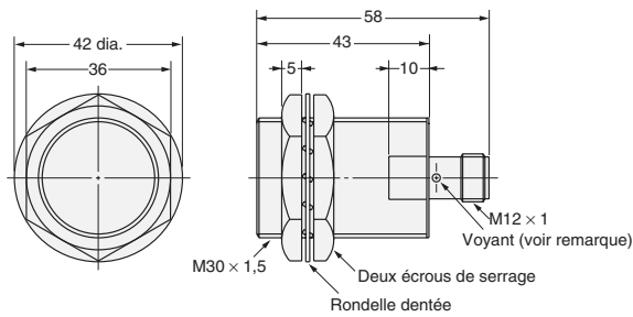
Fig. 13 : E2E-X10Y□-M1
