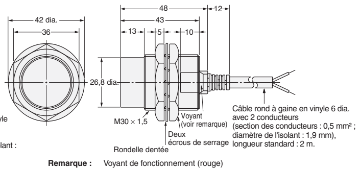
Fig. 8 : E2E-X18MY□
