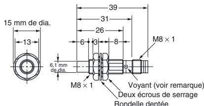
Fig. 28 : E2E-X4MD□-M3G/E2E-X2ME□-M3/F□-M3
