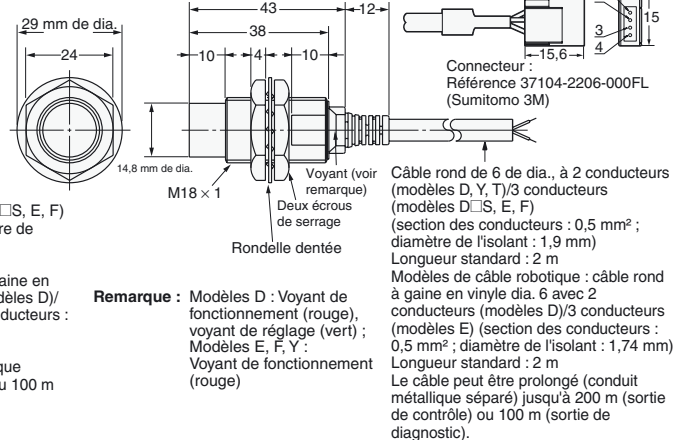
Fig. 16 : E2E-X20MD/ E2E-X18ME-F/ E2E-X18MY
