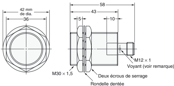
Fig. 25 : E2E-X10D□-M1(G)/E2E-X10E□-M1/F□-M1 E2E-X10Y□-M1
