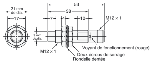
Fig. 24 : E2E-X14MD□-M1(G)/E2E-X10ME□-M1/F□-M1 E2E-X10MY□-M1
