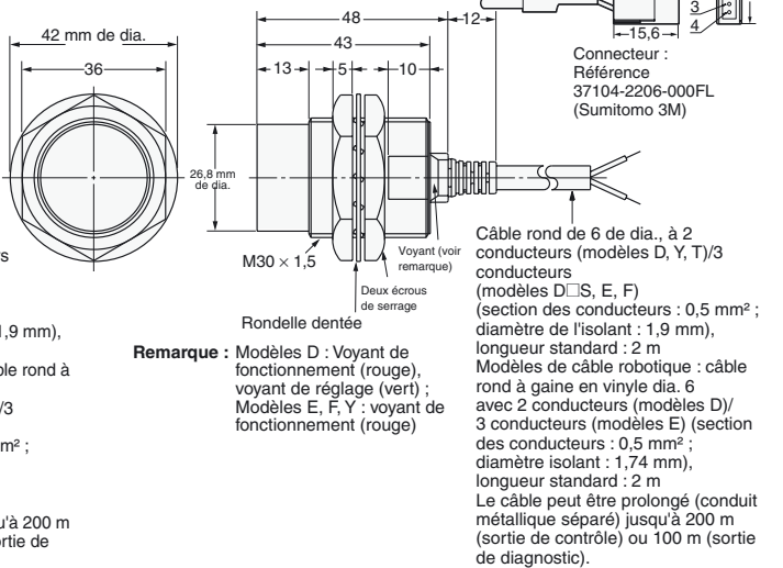
Fig. 16 : E2E-X20MD/ E2E-X18ME-F/ E2E-X18MY
