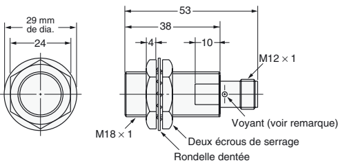
Fig. 23 : E2E-X7D□-M1(G)/E2E-X5E□-M1/F□-M1 E2E-X5Y□-M1
