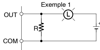
Génération d'un courant d'obscurité (environ 1/3 du courant nominal) dans l'ampoule à incandescence.
