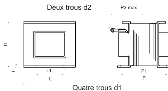
Dimensions externes 2
