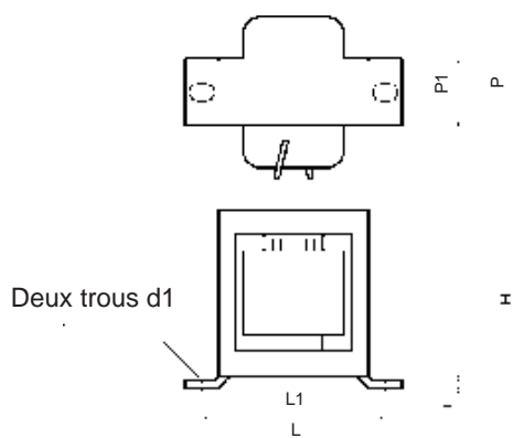
Dimensions externes 1
