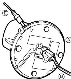
Vue inférieure de la base.
