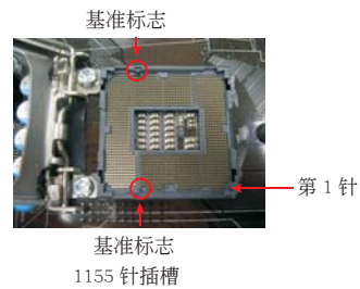
1155 针插槽
