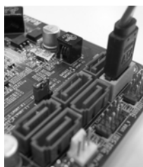
SATAデータケーブルをオレンジSATAIIコネクタ(SATAII_6 (PORT5))に接続します
