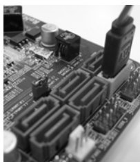
Collegare il cavo dati SATA al connettore SATAII arancione (SATAII_6 (PORT5))
