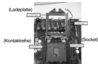
1156-Pin Sockel Übersicht
