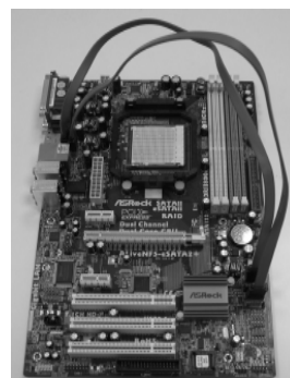
SATAデータケーブルを赤いeSATAIIコネクタ(eSATAII_BOTTOM)とオレンジのeSATAIIコネクタ(eSATAII_TOP)の両方に接続します
