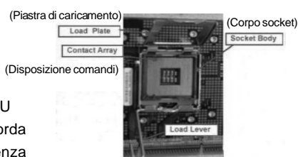
Vista del socket 775-Pin
