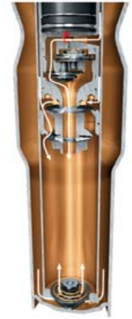
Phase de détente – piston seul = réglage sportif confortable
