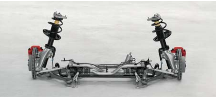
Essieu avant du Boxster S
