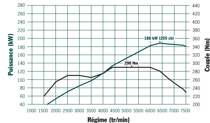
Boxster : 290 Nm entre 4 400 et 6 000 tr/min, 255 ch (188 kW) à 6 400 tr/min
