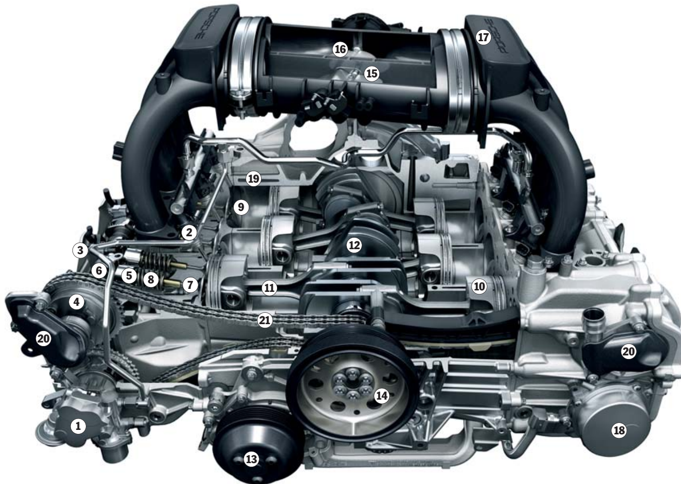
Moteur 6 cylindres Boxer de 3,4 l de cylindrée du Boxster S
