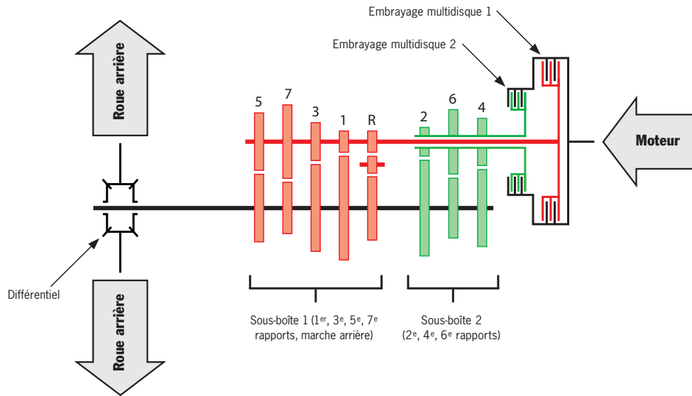
Principe de la boîte de vitesse Porsche Doppelkupplung (PDK)
