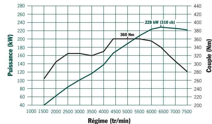
Boxster S : 360 Nm entre 4 400 et 5 500 tr/min, 310 ch (228 kW) à 6 400 tr/min
