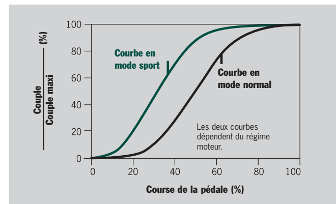
Courbes comparatives de l'accélérateur électronique en mode normal et en mode sport
