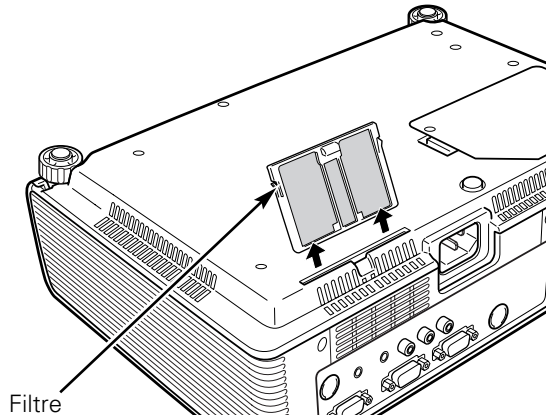
Filtre Retirez en tirant vers le haut.
