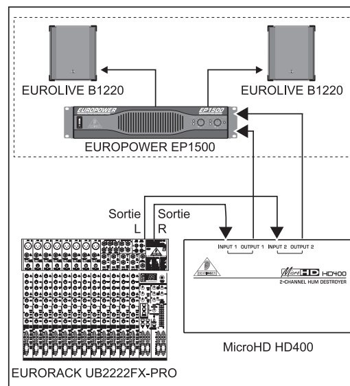
Câblage du HD400
