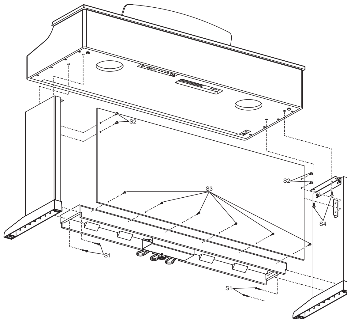
Fig. 2.2 : Montage de l'EG2080
