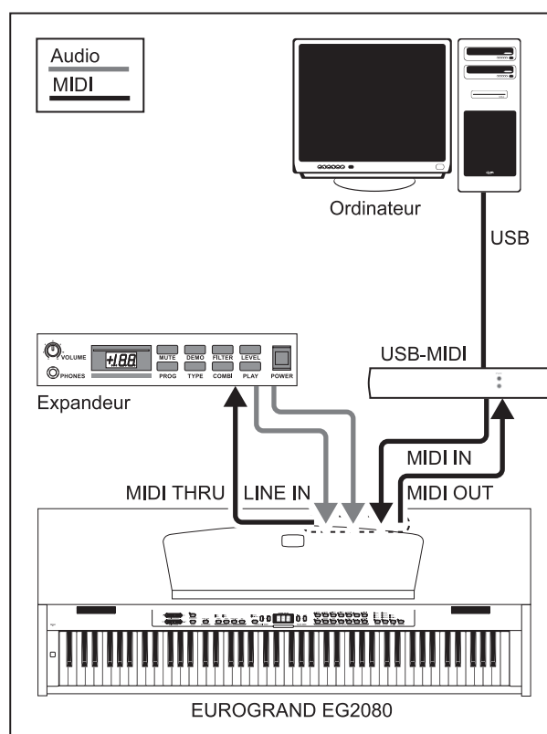
Fig. 7.4 : Système MIDI avec séquenceur logiciel et générateur sonore externe
