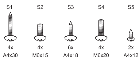
Fig. 2.1 : Eléments et vis de l'EG2080
