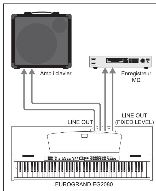
Fig. 7.2 : Câblage avec un ampli et un enregistreur
