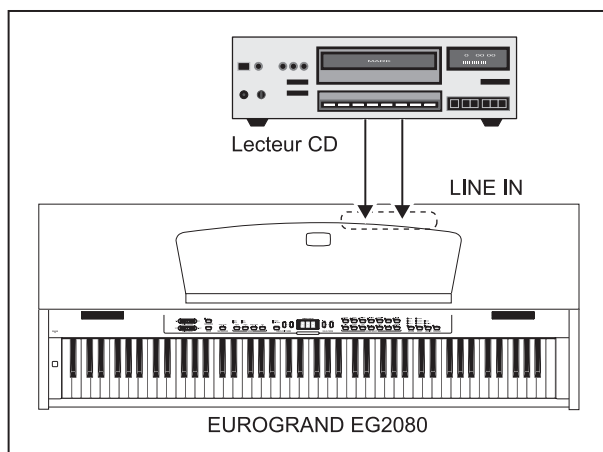
Fig. 7.1 : Câblage de sources externes
