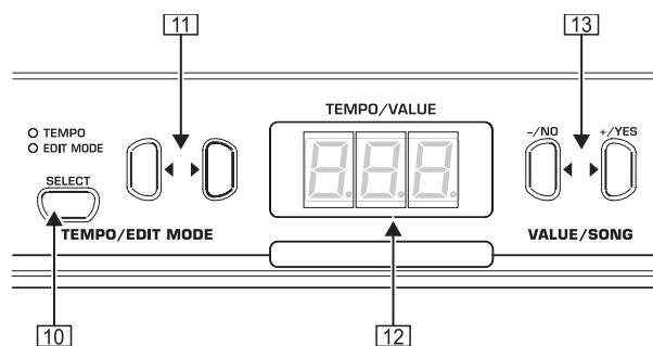
Fig. 4.1 : Commandes de l'EG2080
