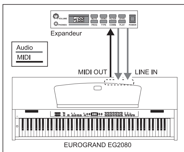
Fig. 7.3 : Commande d'expandeurs MIDI externes
