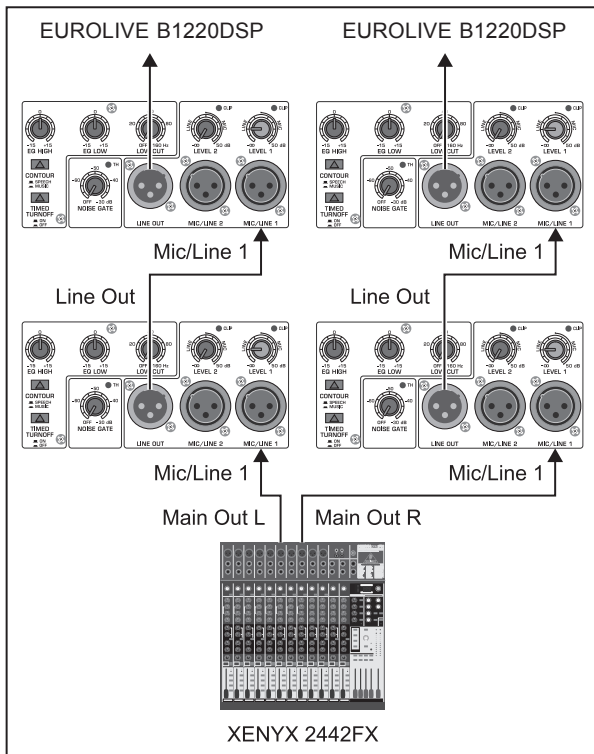
Fig. 3.3 : Chaînage de plusieurs B1220DSP
