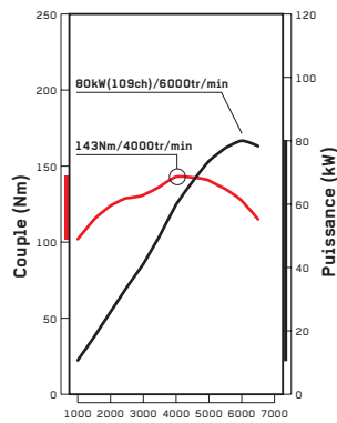
Vitesse du moteur (tr/min) 1.5-litre MIVEC (Non disponible en France)
