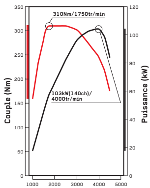
Vitesse du moteur (tr/min) 2.0 litres DI-D
