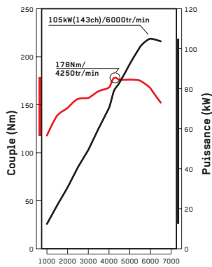
Vitesse du moteur (tr/min) 1.8-litre MIVEC (Non disponible en France)
